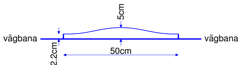
Figure 1: Förslag till nya, permanenta, asfalterade farthinder.
